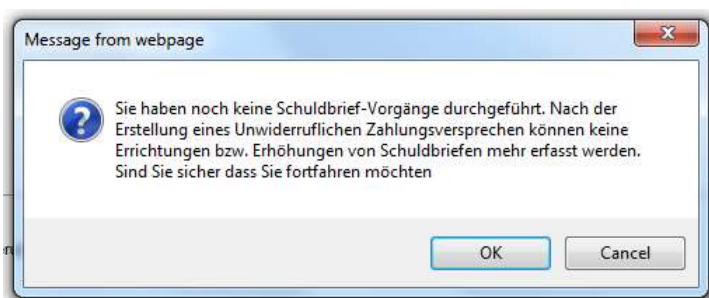
Abbildung 30 - Warnmeldung Zahlungsverprechen
